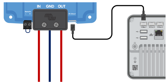
L'Orion XS est piloté par DVCC via un dispositif GX.
