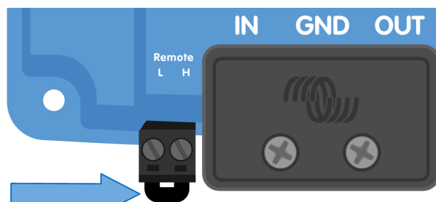
Connecteur d'allumage/arrêt à distance avec boucle de fil
