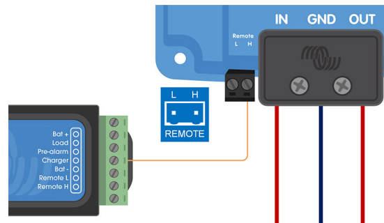
L'Orion XS est piloté par le contact ATC du BMS.
