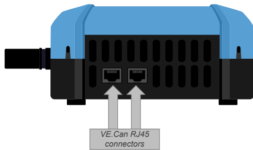
Emplacement des connecteurs VE.Can du Lynx Shunt VE.Can
