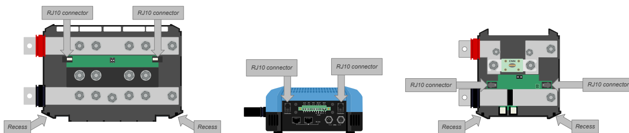
Emplacements des connecteurs RJ10 et des orifices pour câbles RJ10 sur le Lynx Distributor et le Lynx Shunt VE.Can
