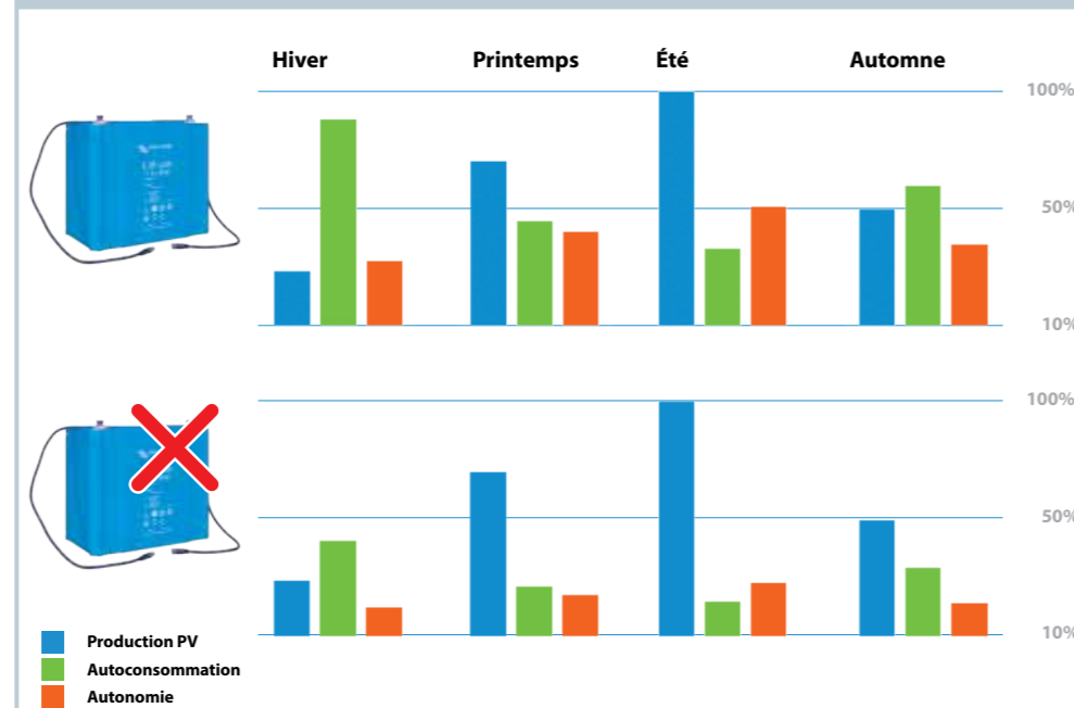
Variations saisonnières types à une latitude d'environ 50 degrés (Seattle, Londres, Amsterdam, Berlin, Munich), avec et sans batterie.
