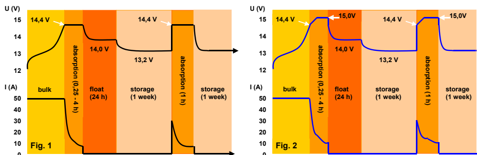
Courbes de charge : jusqu'à la tension de gavage (Fig. 1), et dépassement de la tension de gavage (Fig. 2).
