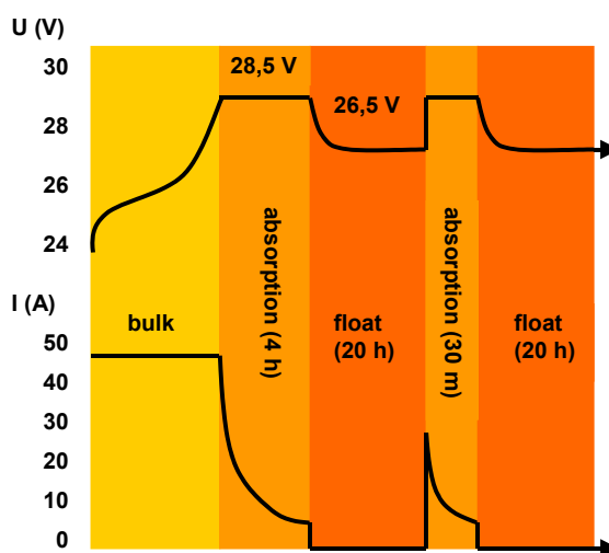
Courbe de charge
